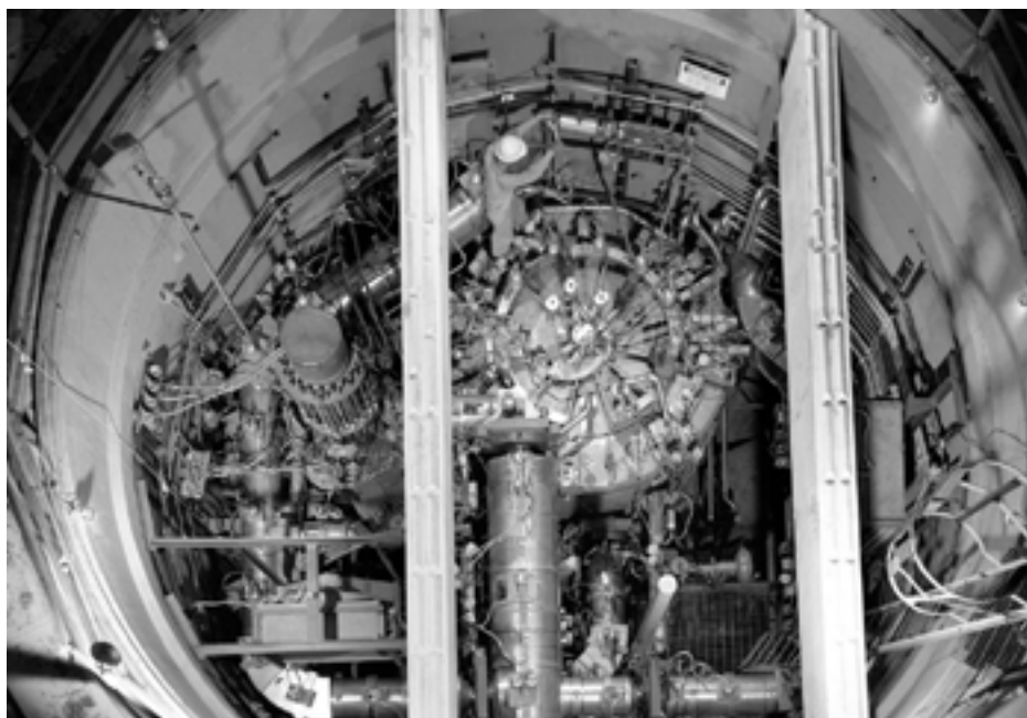
Experimentanläggningen med en toriumreaktor i Oak Ridge National Laboratory. Sedan problem visat sig med saltkylningen var toriumreaktorn näst intill bortglömd i fyrtio år. Nu pågår åter ett intensivt arbete för att undersöka möjligheterna att få billigt torium att ersätta dyrt uran, samtidigt som kostnader och säkerhet förbättras. Observera arbetaren i hjälm högt upp i bildens mitt. Foto: Oak Ridge National Laboratory.
