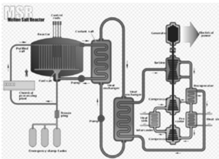
Principskiss för smältsaltreaktor från US Department of Energy Nuclear Research Advisory Committee
