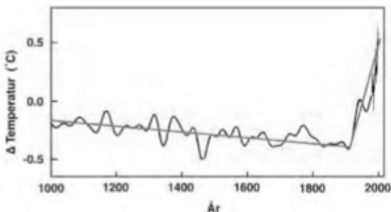
Det beryktade hockeyklubb-diagrammet. En bluff som svaldes av FNs klimatpanel IPCC.
