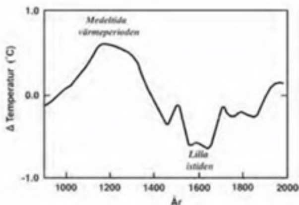
Temperaturutvecklingen sedan år 900
