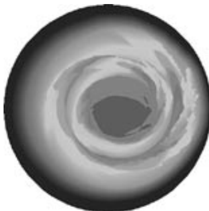
Planeten Mars har blivit varmare sedan 1970-talet.
