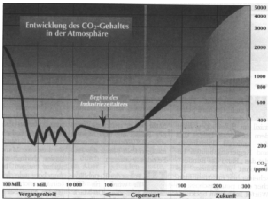
Ett tyskt skräckdiagram där medeltemperaturen går rakt upp i taket. Det är sådana som legat bakom alarmrapporterna om växthuseffekten och Kyoto-protokollet. Men kan man lita på vetenskapen bakom?
