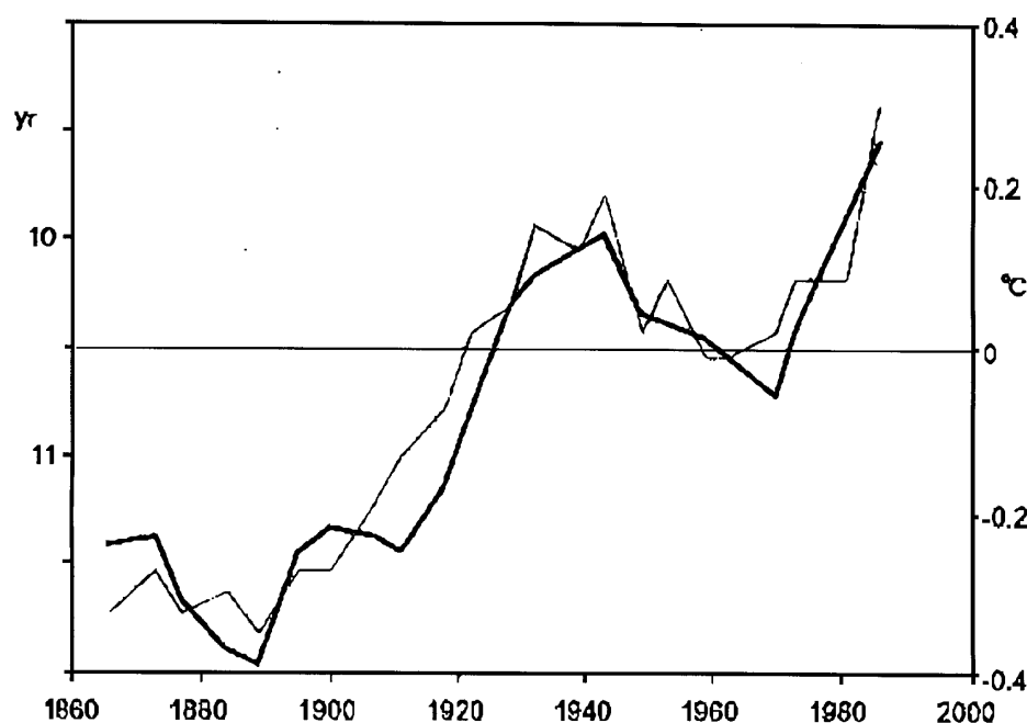
De danska klimatforskarna Eigil Friis-Christensen och Knud Lassen har analyserat sambandet mellan jordens medeltemperatur vid jordytan och solfläckarna. Diagrammet som visar utvecklingen mellan 1865 och 1985 är onekligen talande.
