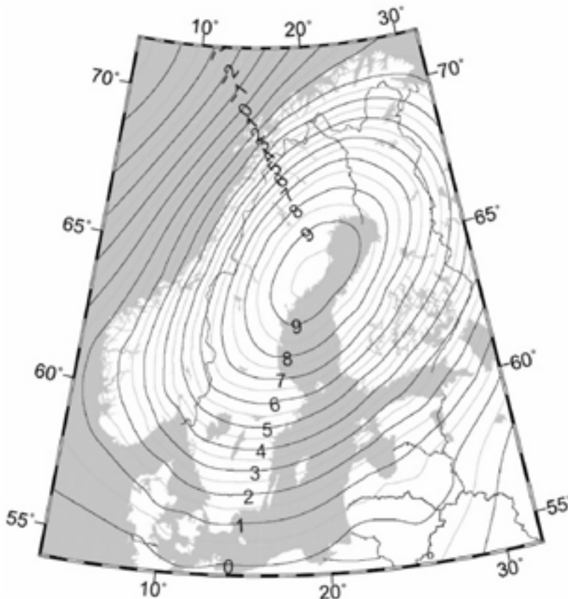
Landhöjning i millimeter per år vid konstant vattenstånd. Först nere vid tysk/polska Östersjö-kusten övergår det i landsänkning. Källa Lantmäteriet.
